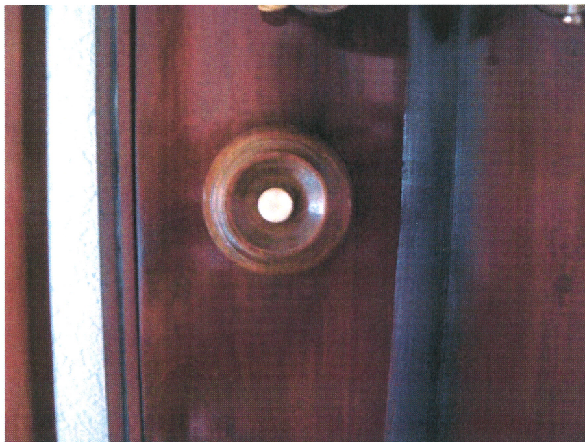
In de kast bevindt zich een knop die bij indrukken na stoomuitval een veer opwindt en zo voor de nodige gangreserve zorgt.
