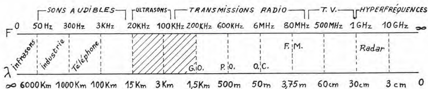
Fig. 2. — Les ondes électromagnétiques se caractérisent par leur fréquence F ou leur longueur d'onde \lambda . Les zones hachurées sont celles utilisées pour la transmission des signaux horaires.
