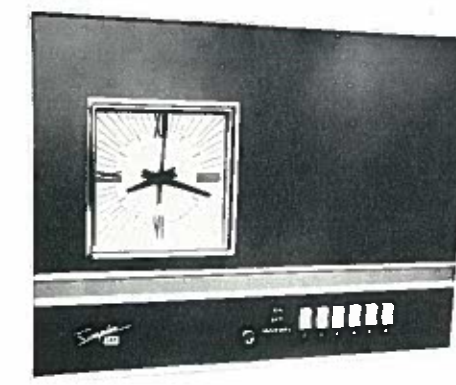
Quarzhauptuhr mit Programm- Einrichtung für 6 Kreise Type 93
