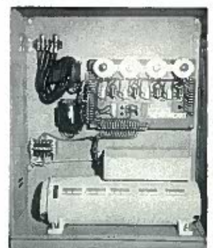
Sender-Generator 1000 VA für elektronische Uhren- und Steueranlage
