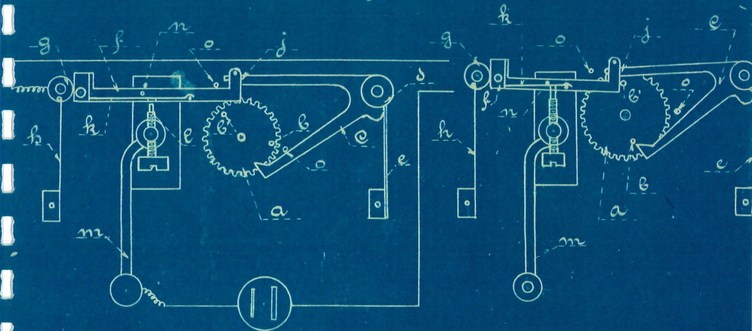
Dispositif du contact de la pendule mère.
