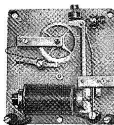
Mouvement Récepteur n° 2
