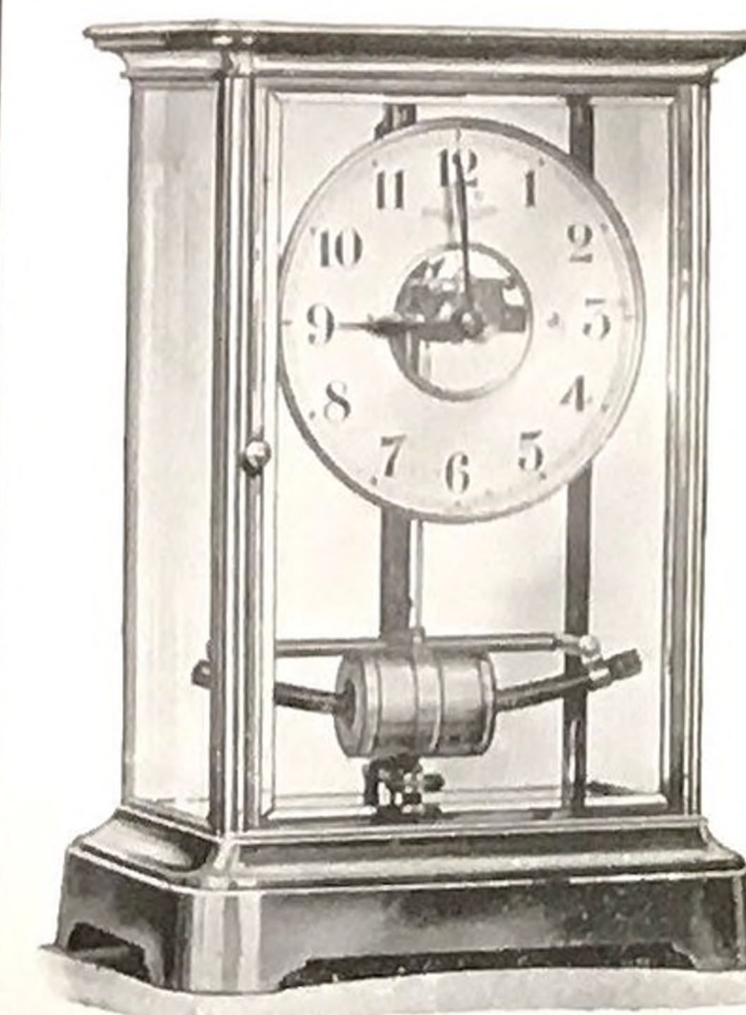
N° 5. — H. — Régulateur bronze patiné or, 4 glaces biseautées (succès mondial). Hauteur 34 cm. Balancier long. 10 cm. 5. Prix imposé 660 Le même en chrome inaltérable 735
