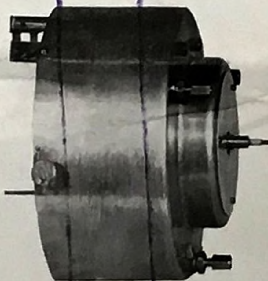
Ensemble (sans balancier) du nouvel emboîtement "BULLE". Diamètre total 98 m/m. Hauteur — 80 m/m.
