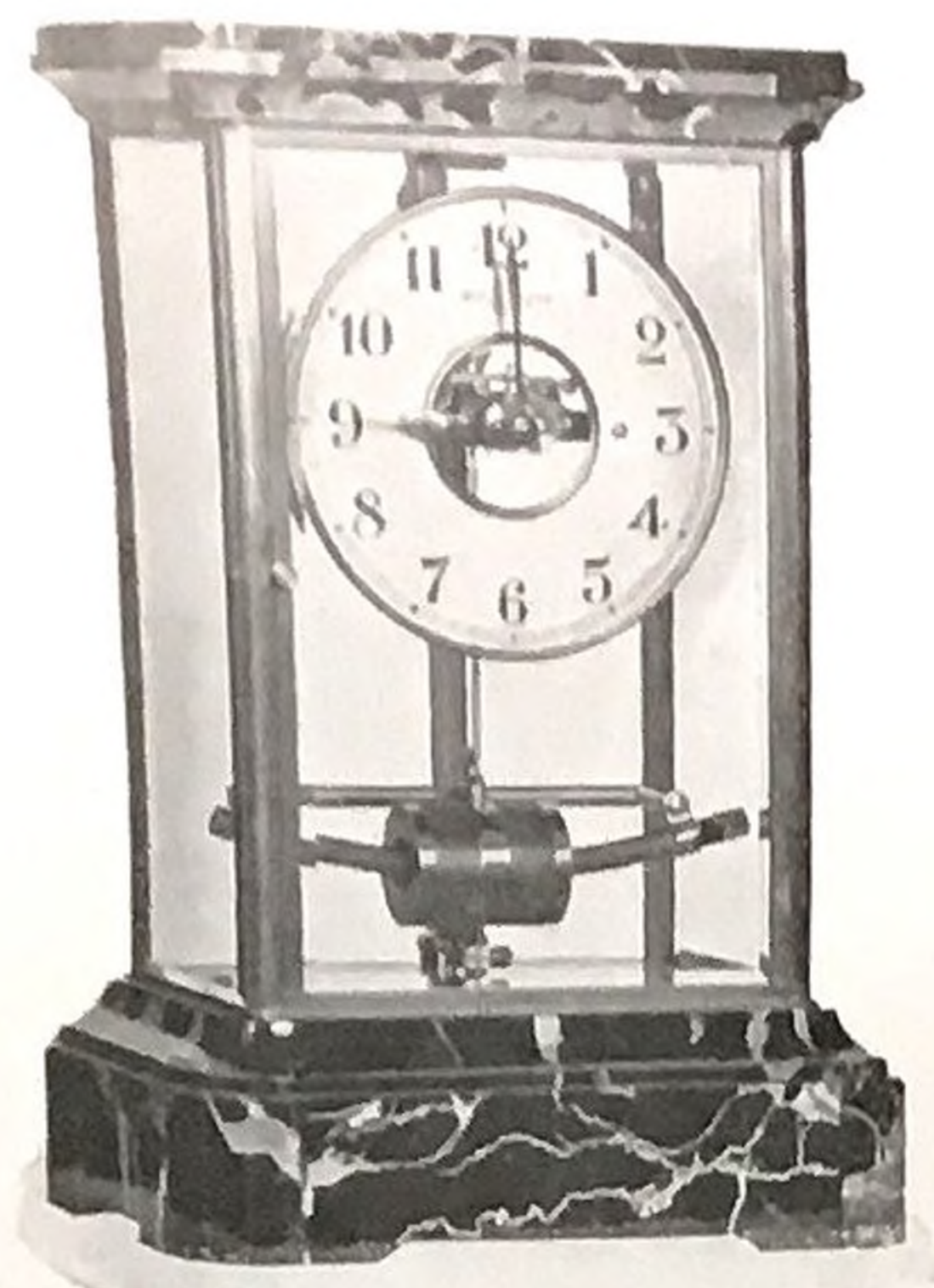
N° 1. — L. — Régulateur 4 glaces biseautées, montants bronze patiné or mat, socle et chapiteau marbre. Se fait en vert de mer, skyros, griotte, porior, onyx d'Algérie, jaune de Sienné. Hauteur 37 cm. 5. Balancier long. 24 cm. 5. Prix imposé 800
