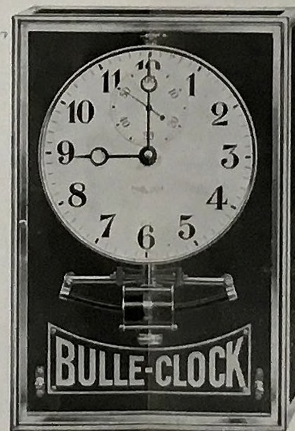
N° 15. — Z. — "LE GARDE TEMPS". Régulateur de haute précision. Cabinet en bronze chromé, 5 glaces biseautées. Hauteur 38 cm. Largeur 26 cm. Balancier long. 29 cm. 5. Prix imposé 1700
