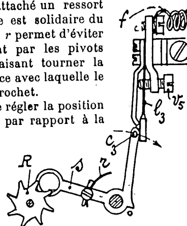
FIG. 8. — Détails du contact entretenant les oscillations.
