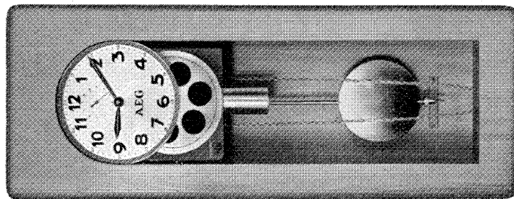
Bild 3. Hauptuhr mit \frac{3}{4} -Sekundenpendel
