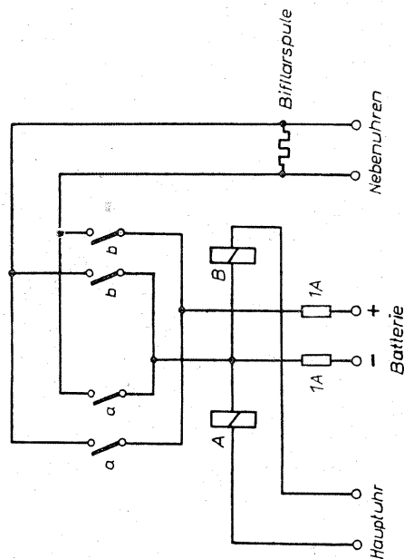
Reihenfolge der Klemmen von vorn gesehen Bild 11. Schaltplan des polarisierten Zwischenrelais
