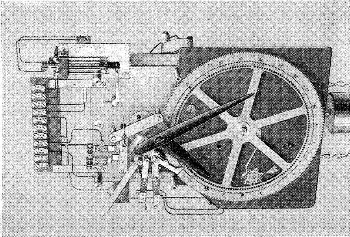
Bild 6. Vorderansicht des Hauptuhrwerkes mit Signaleinrichtung
