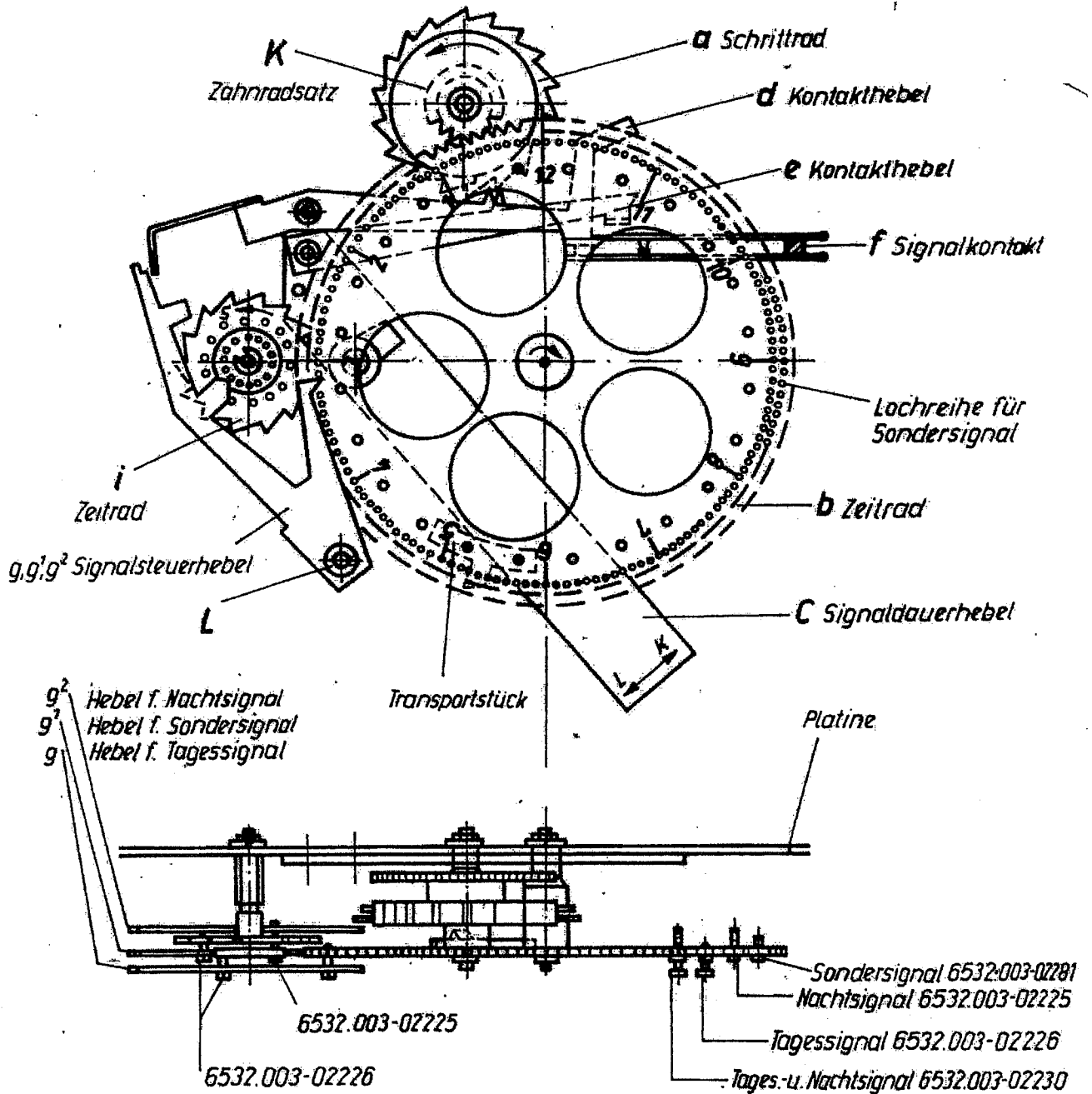
Signaleinrichtung
